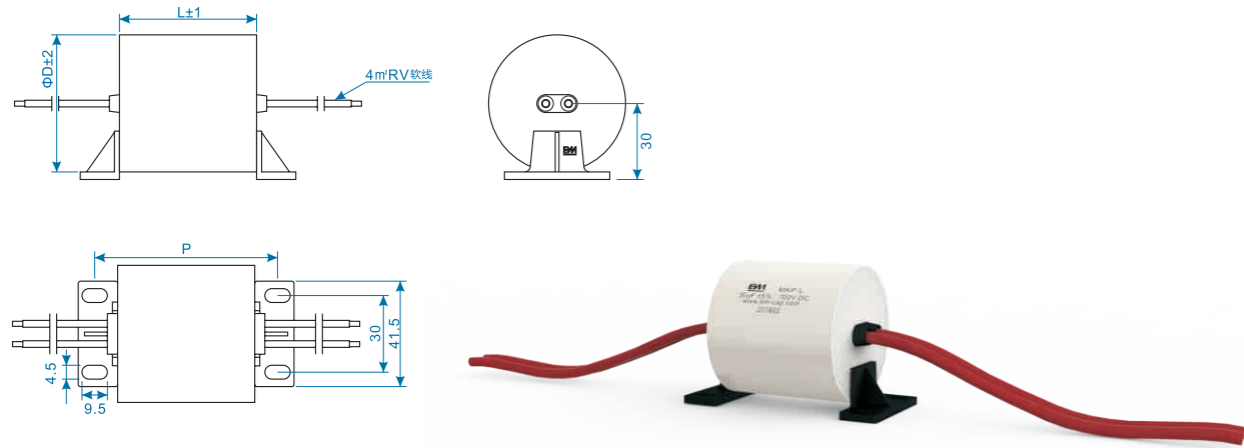
C类结构 C Class
