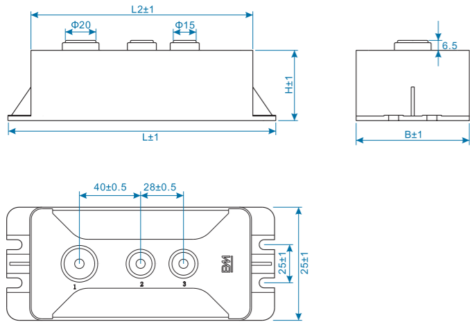
A类结构 A Class
