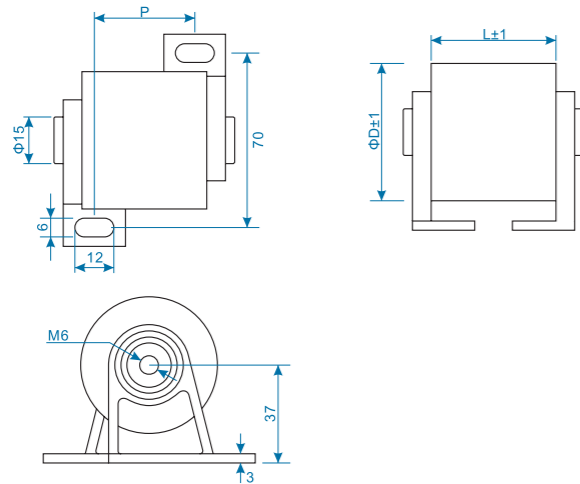
B类结构 B Class
