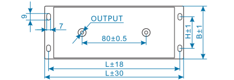
常用规格 Dimension
