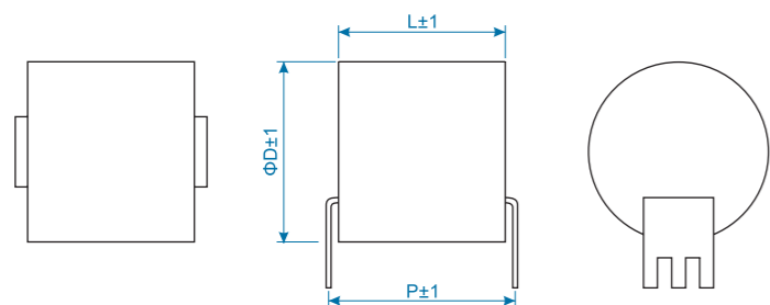
A类结构 A Class
