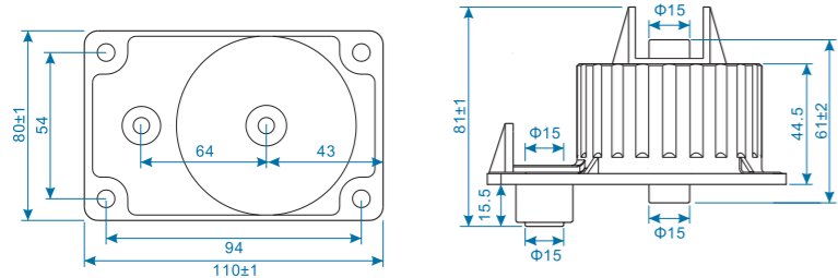
B类结构 B Class
