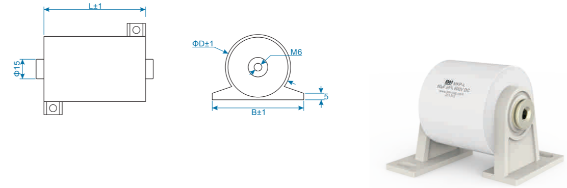
E类结构 E Class
