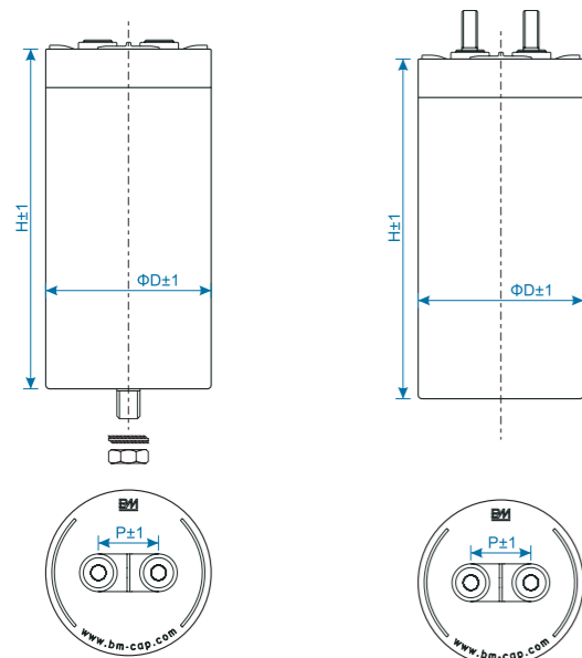
接线方式 Connection M6铜螺母 安装方式 Installation M12螺栓 接线方式 Connection M8铜螺栓 安装方式 Installation 平底
