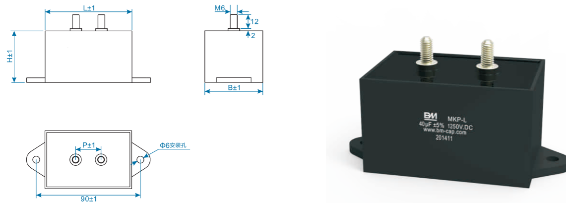
D类结构 D Class
