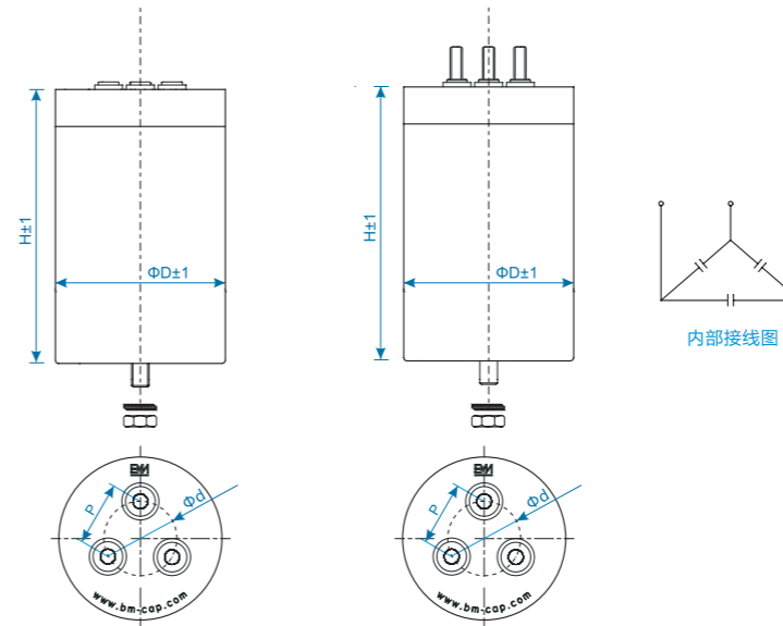
接线方式 Connection M6铜螺母 安装方式 Installation M12螺栓 接线方式 Connection M8铜螺栓 安装方式 Installation M12螺栓
